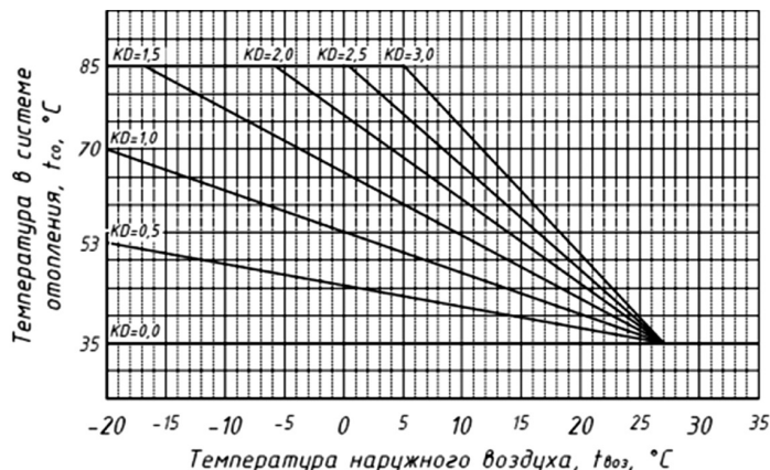
Рис. 9. Кривые нагрева
